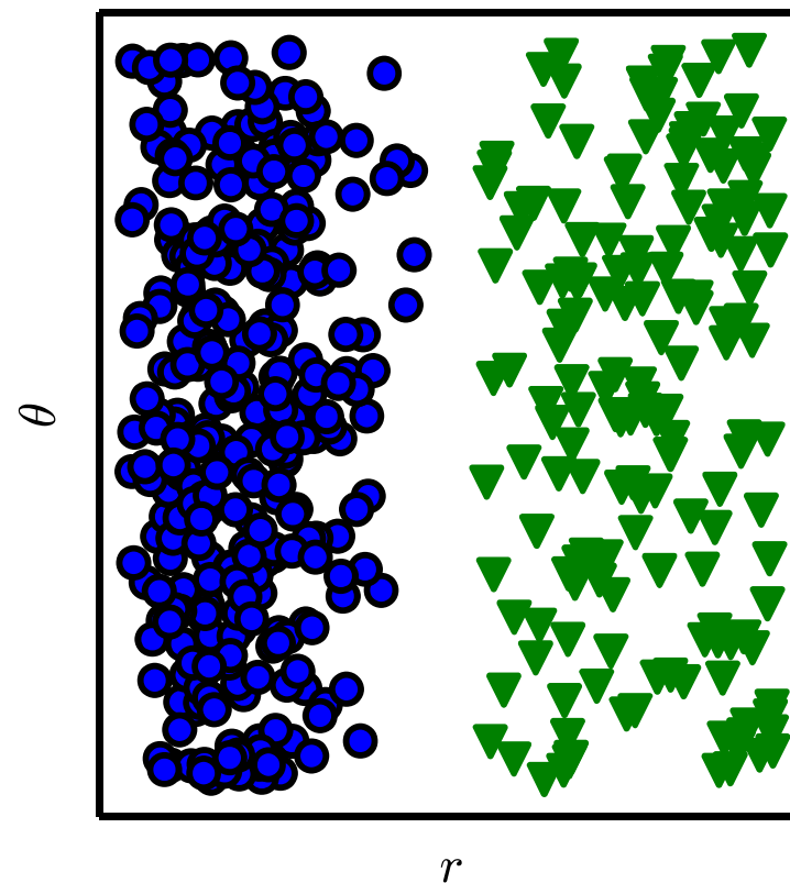
Polar coordinates
